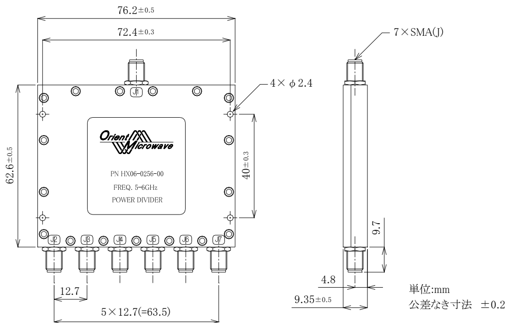
外形図
