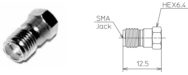
■SMAジャック SMA Jack 許容電力は25℃時0.5W Power watts avg: 0.5W @25℃
