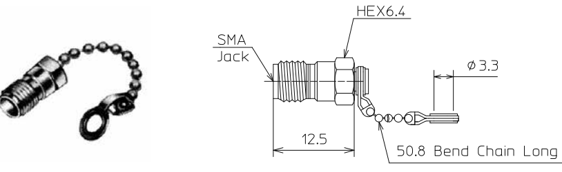
■SMAジャックチェーン付 SMA Jack With Chain 許容電力は25℃時0.5W Power watts avg: 0.5W @25℃
