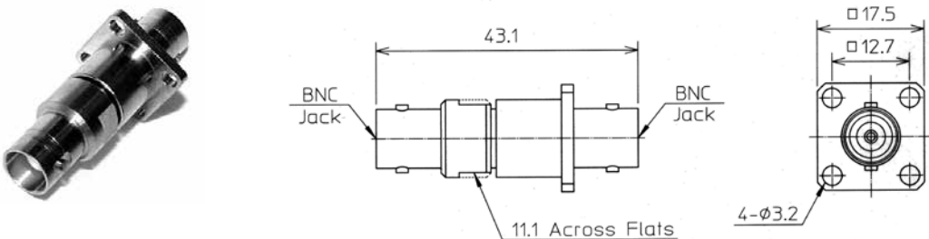
■BNCジャックーBNCジャック BNC Jack - BNC Jack
