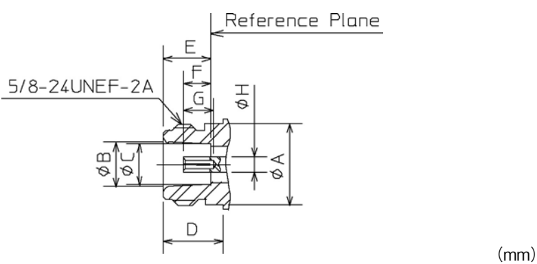
ジャック Jack
