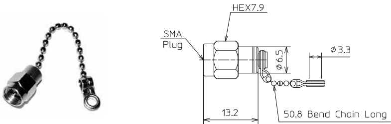
■SMAプラグチェーン付 SMA Plug With Chain 許容電力は25℃時1W Power watts avg: 1W @25℃
