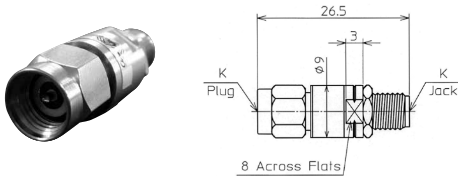
Kプラグージャック【耐電力 25℃時 1W】 K plug - jack [withstanding power at 25℃: 1W]
