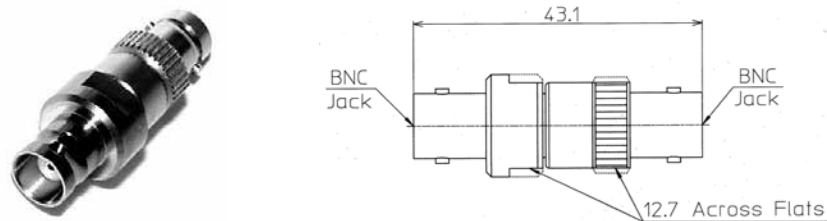
■BNCジャックーBNCジャック BNC Jack - BNC Jack
