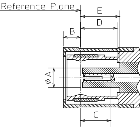
フィメー ル Female
