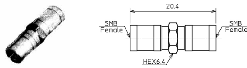
■SMBフィメールーSMBフィメール SMB Female - SMB Female
