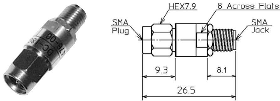
SMAプラグージャック【耐電力 25℃時 2W】 SMA plug - jack [withstanding power at 25℃: 2W]
