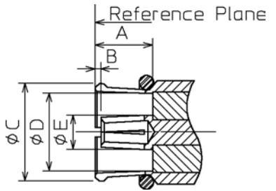
ジャック Jack
