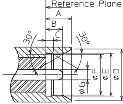
プラグ (ロック) Plug (Lock)
